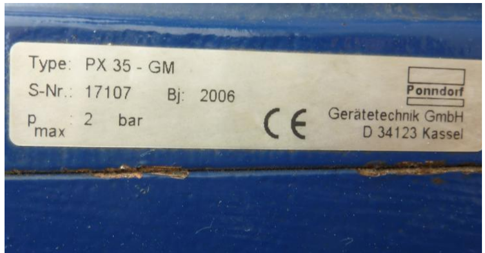
Ponndorf Pumpe
