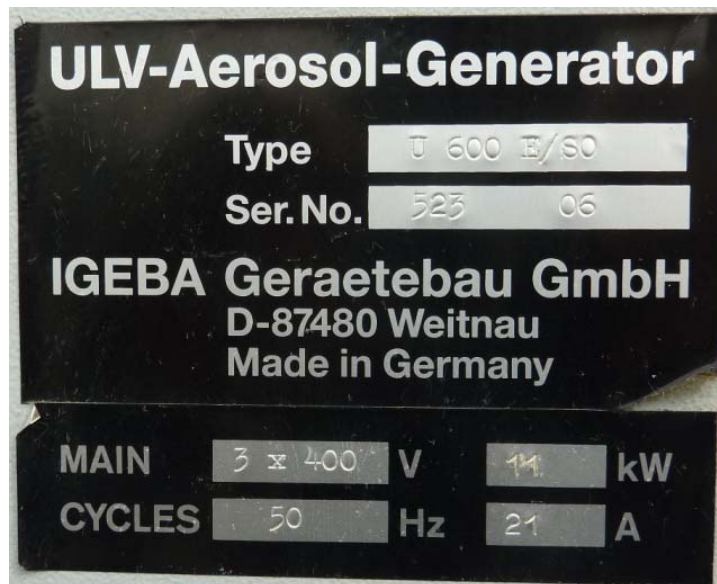
Igeba ULV-Aerosol-Generator
